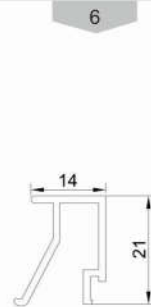
زهوار دو جداره Double rickety Code : 12351 weight : 0.22 kg/m
