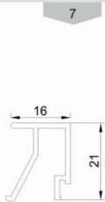
زهوار دو جداره Double rickety Code : 12352 weight : 0.23 kg/m
