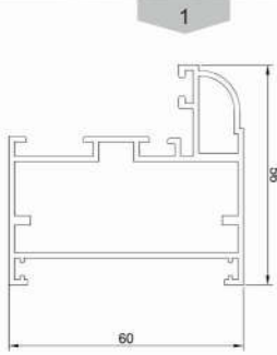
پروفیل فریم Frame profile Code : 13311 weight : 1.14 kg/m
