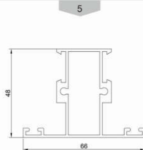
پروفیل سپری T profile Code : 13341 weight : 1 kg/m
