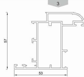
پروفیل لنگه پنجره Vent profile Code : 13331 weight : 1.11 kg/m
