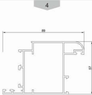
پروفیل لنگه درب Vent profile Code : 13332 weight : 1.3 kg/m
