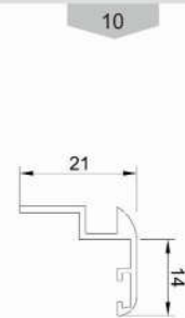
روکوب ۱۴ Suppressed the binding Code : 10021 weight : 0.2 kg/m
