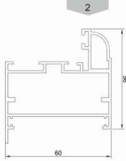
پروفیل فریم Frame profile Code : 13312 weight : 1.17 kg/m
